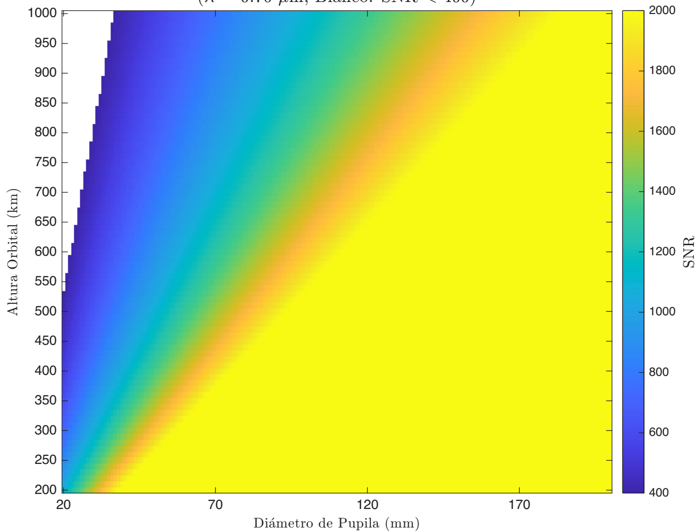
SNR - Korsch - Detector 3 ( \lambda = 0.76 \mu\text{m} , Blanco: SNR < 400)
